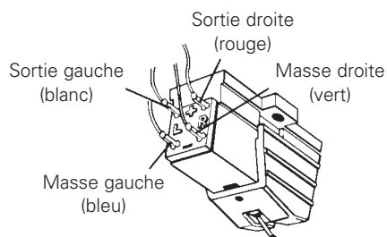
Figure 8 – Branchements électriques
