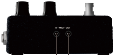
MIDI IN / OUT接口
